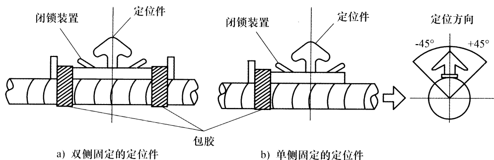
图7 定位件安装示意图
