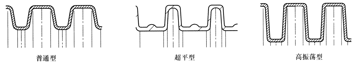
图 D.1 波纹管波形结构示意图
