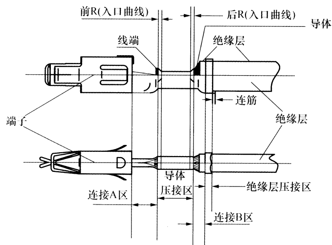
图9 端子与电线连接示意图
