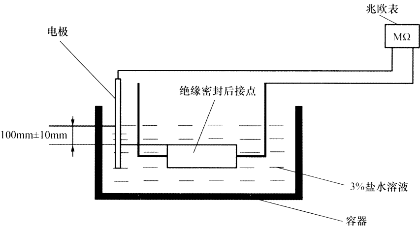
图 18 接点浸水试验示意图
