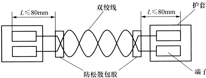
图 5 插接器部位包胶尺寸示意图
