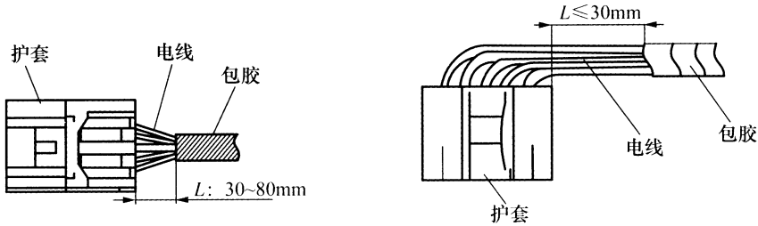
图 5 插接器部位包胶尺寸示意图
