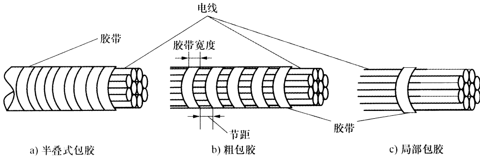
图3 包胶方式示意图
