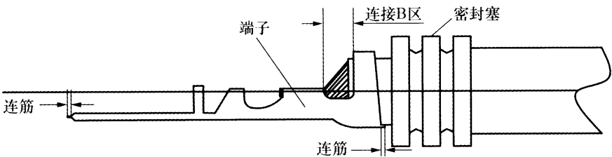
图 11 带密封塞绝缘压接示意图
