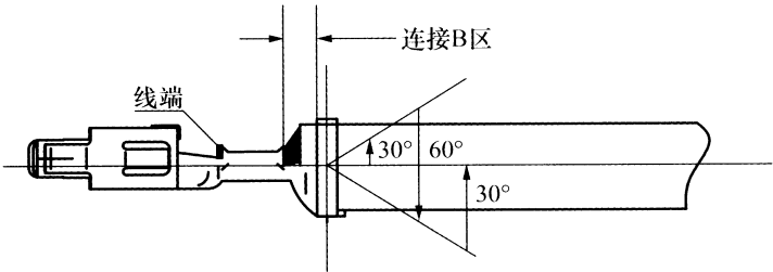
图 10 绝缘层压接示意图
