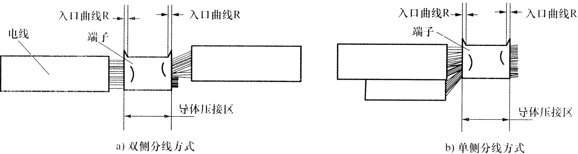
图 12 压接接点示意图
