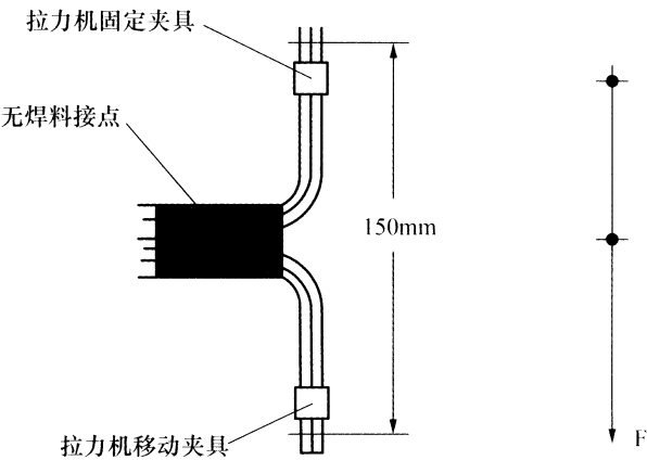
图 19 撕裂力试验示意图
