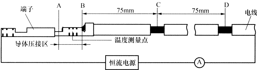
图 16 电压降试验示意图
