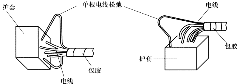
图4 插接器部位包胶示意图
