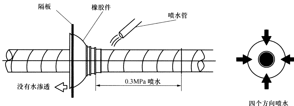
图 20 橡胶件防水密封试验示意图
