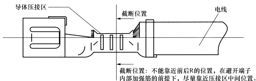
图 15 截断位置示意图
