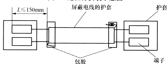
图7 定位件安装示意图
