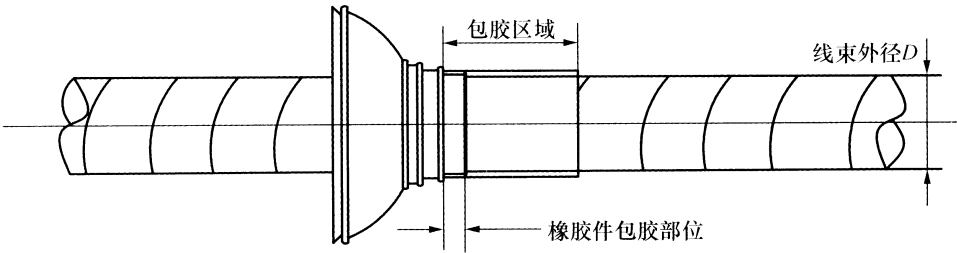
图 14 橡胶件安装示意图
