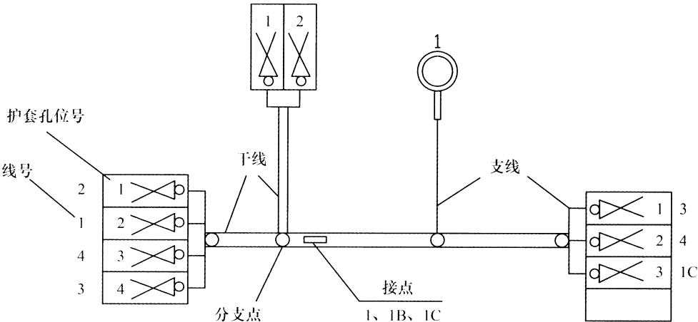
图 1 电线束示意图
