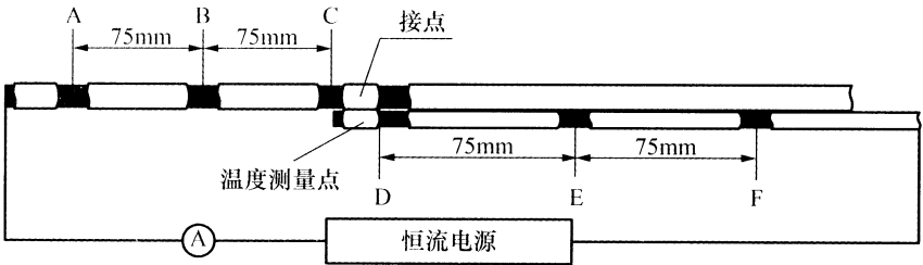
图 17 压接接点电压降试验示意图
